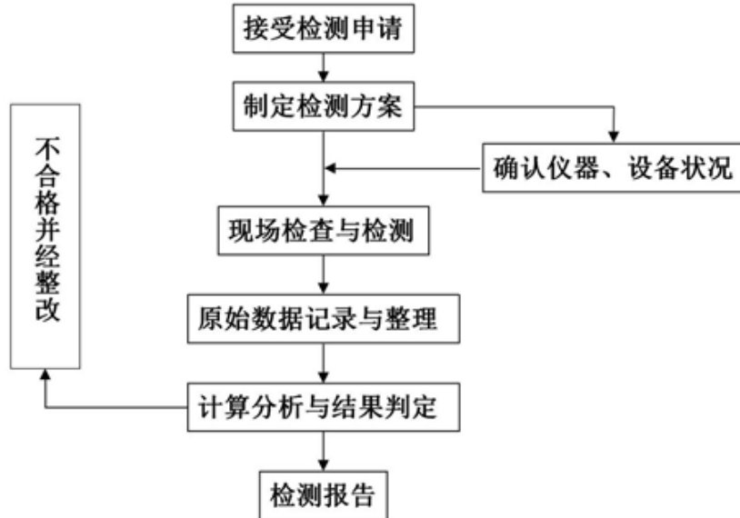
图 B.1 防雷装置检测工作程序框图
