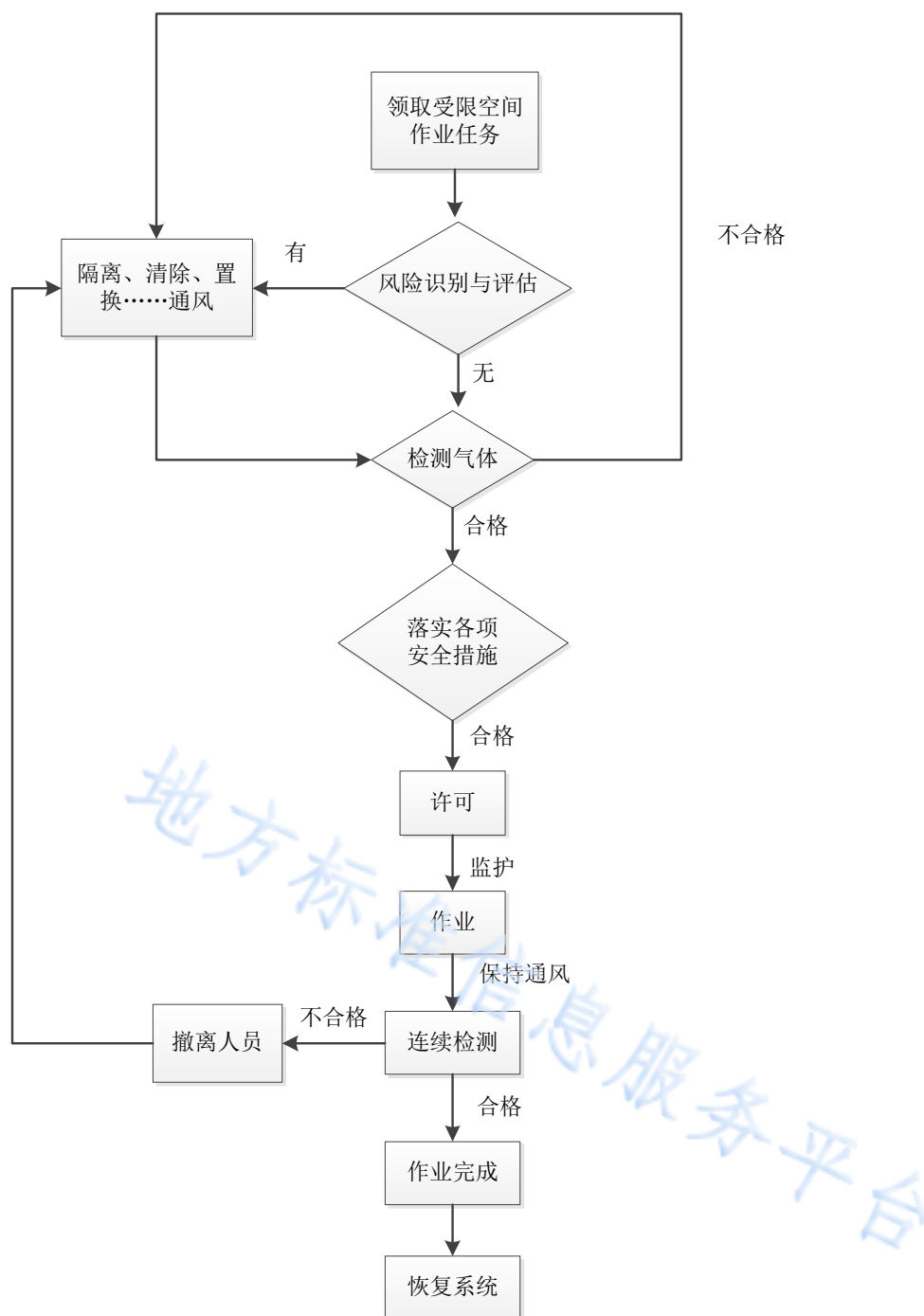
图A.1 进入受限空间危险作业流程
