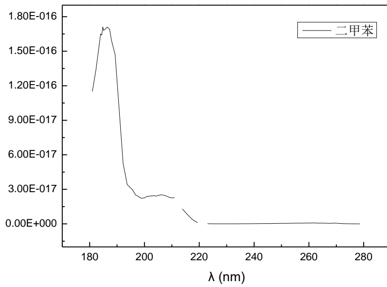
图C.5 二甲苯的紫外吸收光谱
