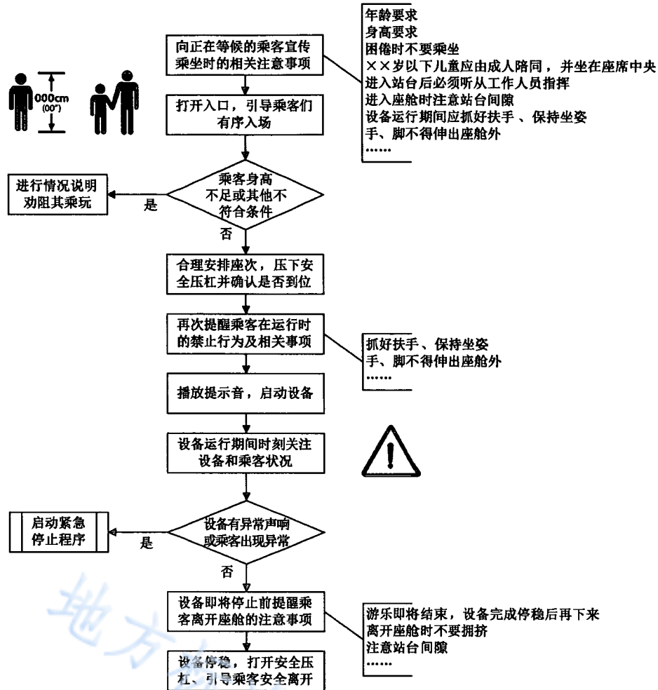
B.1 图 B.1 为某旋转类游乐设施正常运行情况下的操作程序示例。
