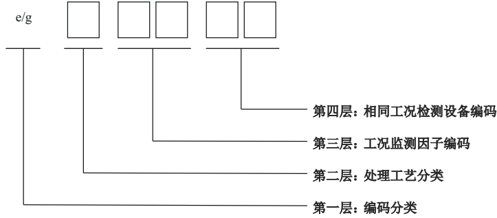
图 B.2 工况监控因子编码规则
