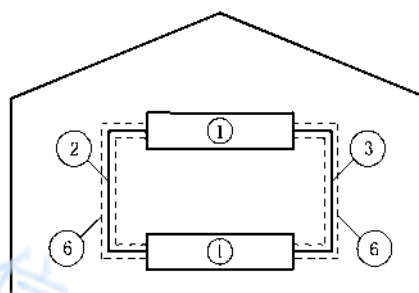
b) 用空间屏蔽减小LPZ内部磁场
