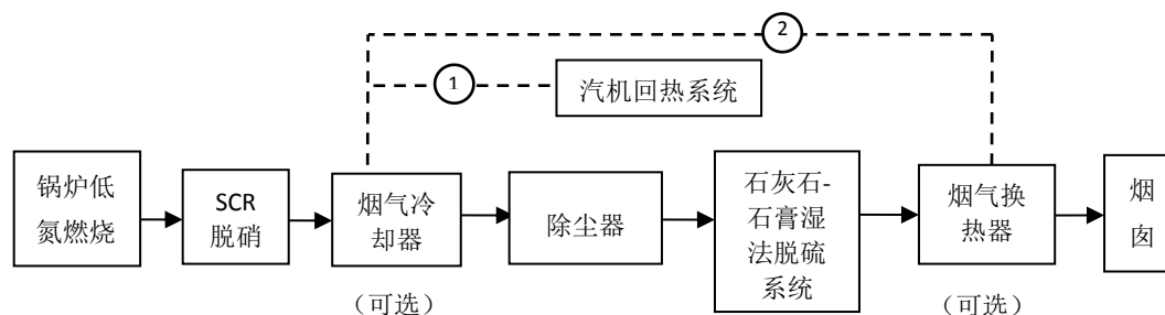
图 E.2 以湿法脱硫协同高效除尘作为二次除尘的典型超低排放技术路线
