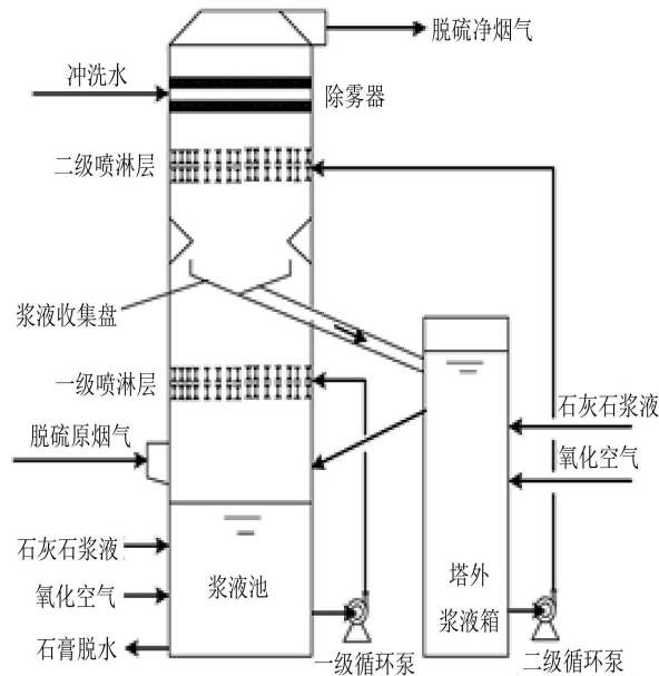
图 G.1 典型石灰石-石膏湿法 pH 值物理分区双循环脱硫工艺流程
