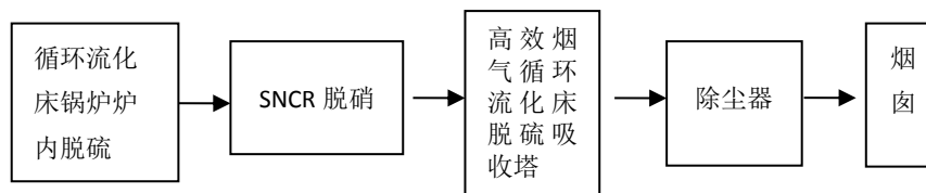
图 E.4 以高效烟气循环流化床作为炉后脱硫工艺的循环流化床锅炉典型超低排放技术路线
