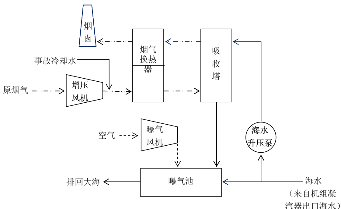
图1 典型海水法烟气脱硫工艺流程示意图
