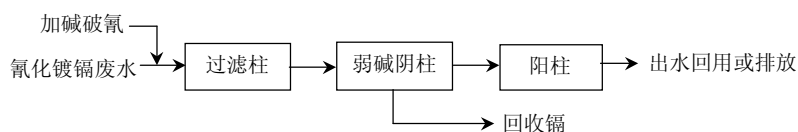
图 9 氰化镀镉废水离子交换处理基本工艺流程
