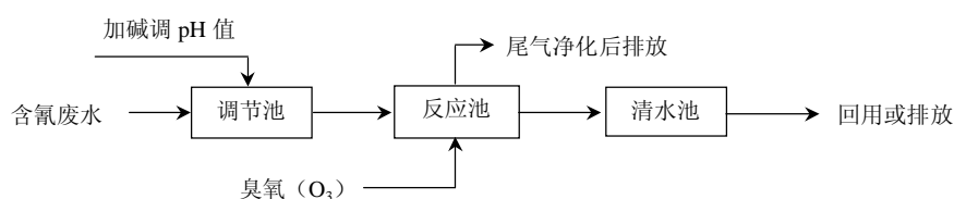
图 2 臭氧氧化处理含氰废水基本工艺流程
