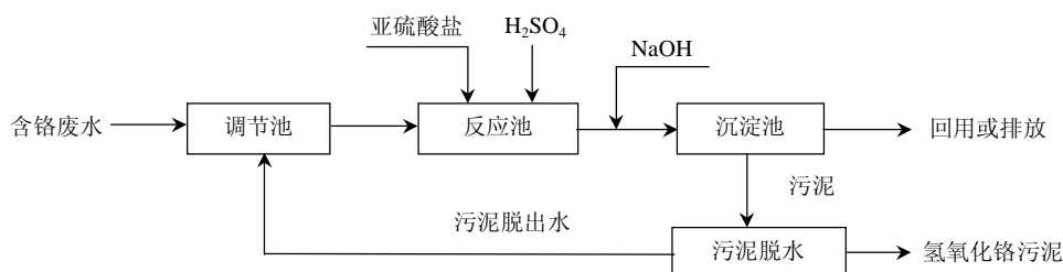
图 4 亚硫酸盐还原处理含铬废水基本工艺流程
