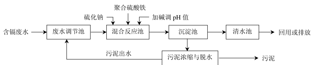
图 8 硫化物沉淀处理含镉废水基本工艺流程
