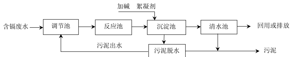
图7 化学沉淀处理含镉废水基本工艺流程
