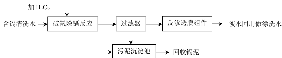
图 11 化学沉淀-反渗透联合处理氰化镀镉废水基本工艺流程
