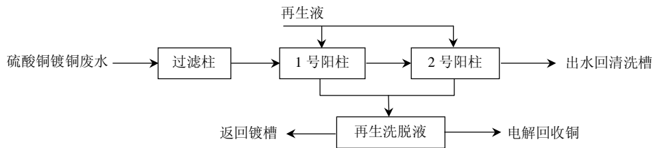
图 15 离子交换处理硫酸铜镀铜废水基本工艺流程
