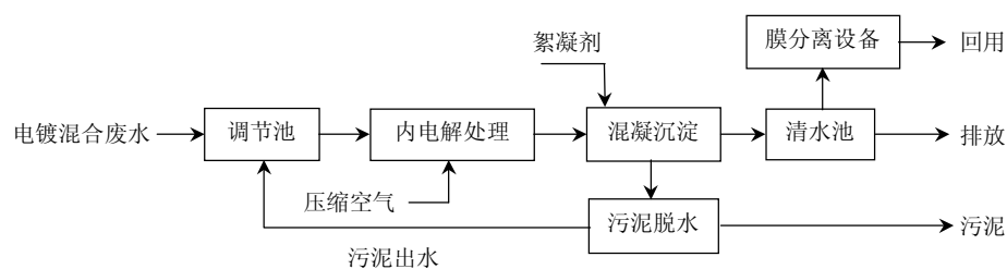
图 23 微电解-膜分离联合处理含铬废水基本工艺流程
