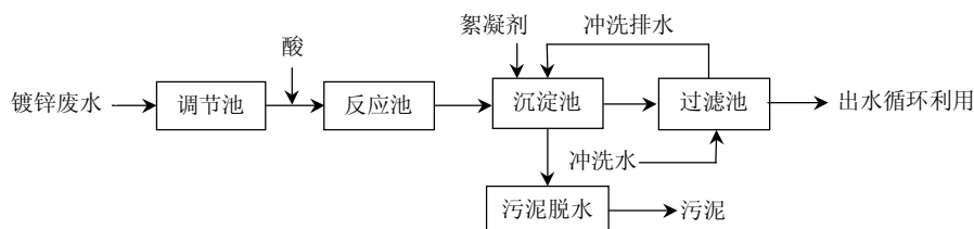
图 18 化学沉淀处理碱性锌酸盐镀锌废水基本工艺流程
