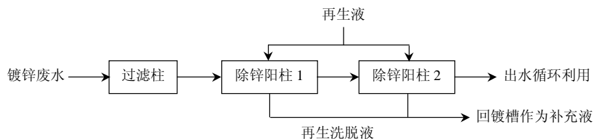
图 20 离子交换处理钾盐镀锌废水基本工艺流程
