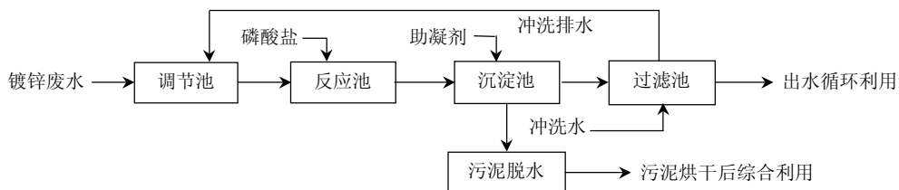
图 21 磷酸盐沉淀处理含铅废水基本工艺流程
