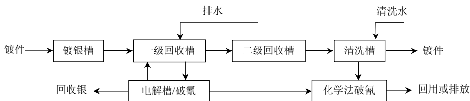
图 22 镀银废水处理基本工艺流程
