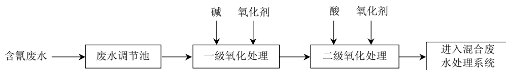
图 1 碱性氯化处理含氰废水基本工艺流程
