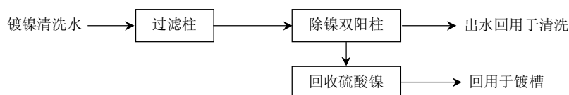
图 12 离子交换处理镀镍清洗水基本工艺流程
