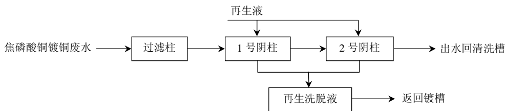
图 16 离子交换处理焦磷酸铜镀铜废水基本工艺流程
