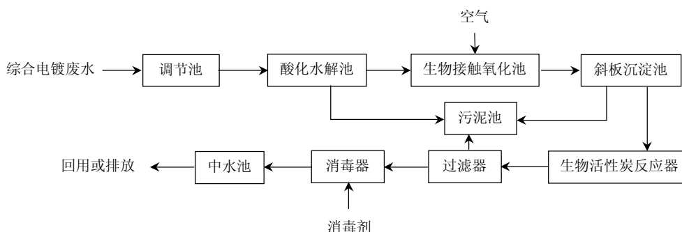
图 24 生物处理综合电镀废水基本工艺流程
