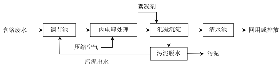
图 5 微电解处理含铬废水基本工艺流程
