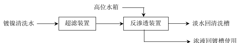
图 13 反渗透处理含镍清洗水基本工艺流程
