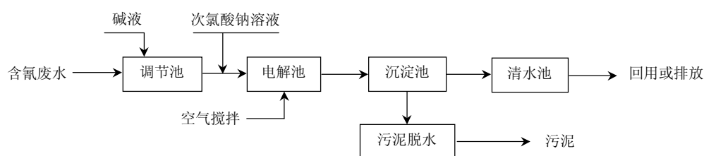
图 3 电解处理含氰废水基本工艺流程
