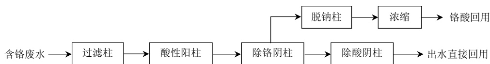
图6 离子交换处理含铬废水基本工艺流程
