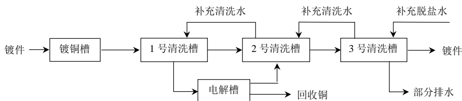
图 17 电解处理镀铜废水基本工艺流程
