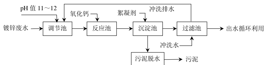
图 19 化学沉淀处理铵盐镀锌废水基本工艺流程
