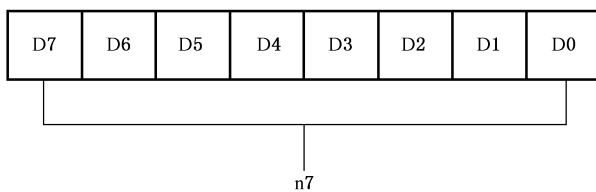
图 A.12 分字节格式
