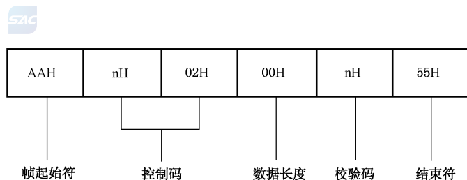
图 A.13 请求帧(3)格式
