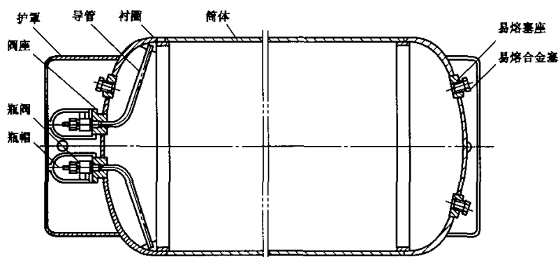
图 2 焊接气瓶结构示意图
