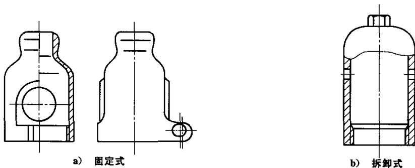
图 7 瓶帽形状示意图
