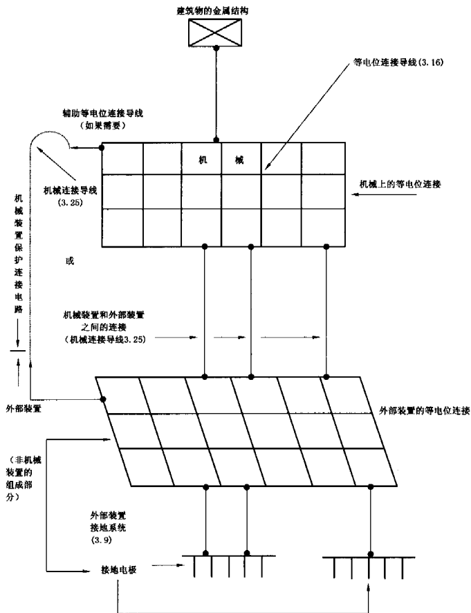
图 2 机械的电气设备等电位连接示例(见 3.15)
