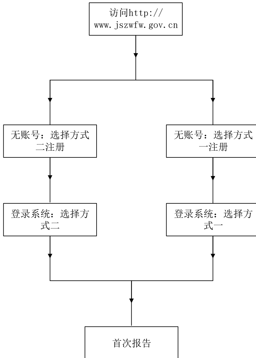
图 0-1 系统流程
