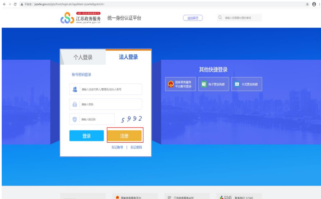
图 0-6 法人注册
