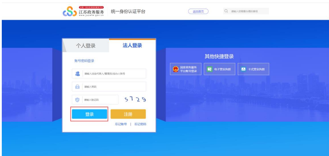
图 0-4 登录
