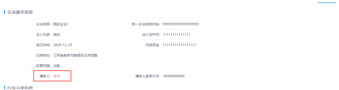
图 0-2 被修改内容
