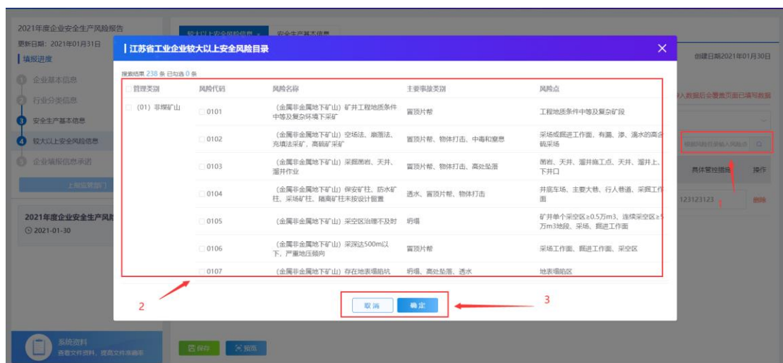
0-8 风险选择
