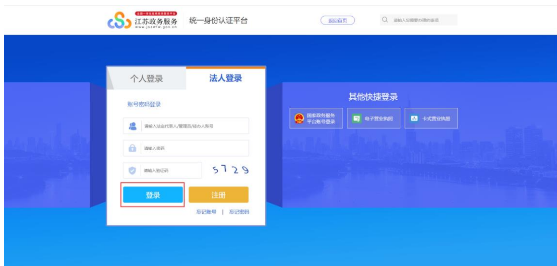
图 0-2 法人登录
