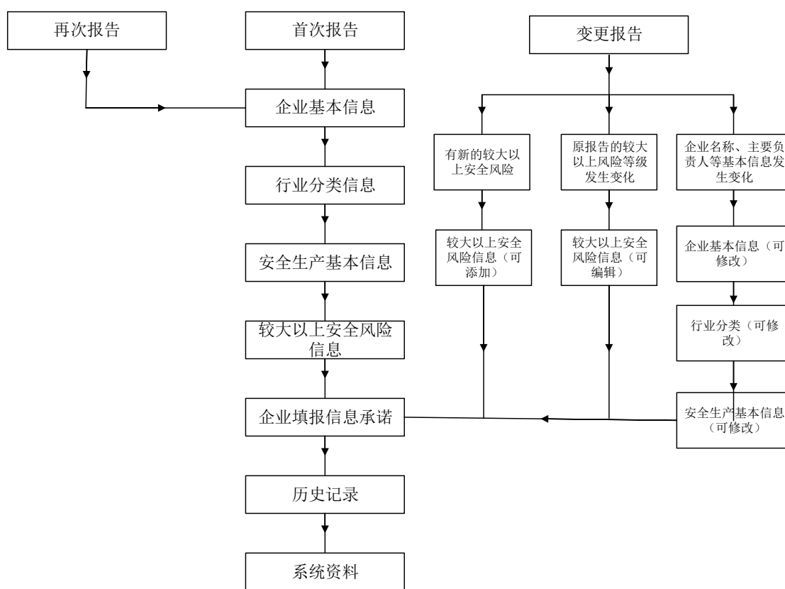
图 0-1 系统流程
